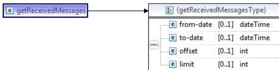
Pav. 1. getReceivedMessages metodo iškvietimo parametrai
