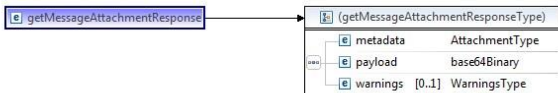
Pav. 14. getMessageAttachment metodo gražinamas rezultatas
